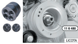
Специальный инструмент для проворачивания коленчатого вала BMW (2.5D/3.0D) ATA-4405
