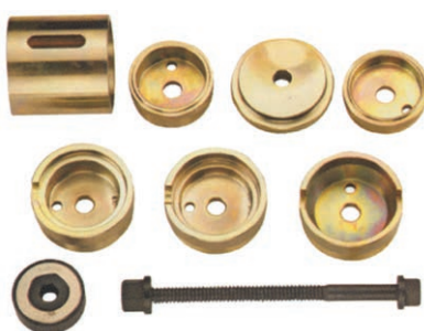
Приспособление для замены сайлентблоков Mercedes ATC-2204
